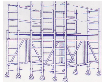
3 x Typ KL 07-20-17 best. aus 2 oder mehr Verbindungsbünnen – breitseitiger Aufbau – beliebig erweiterbar (gleicher Aufbau auch mit Typ KL 13-20-17 möglich)
