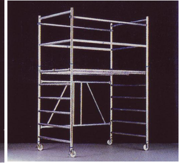
Typ KL 13-20-17 Maße: B 1,30 x L 2,10 x H 2,75 m, Arbeitsbühnenfläche B 1,20 x L 2,00 m, Gewicht 63 kg, Standhöhe 1,70 m
