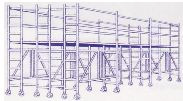
6 x Typ KL 07-20-17 best. aus 9 oder mehr Verbindungsbünnen – längsseitiger Aufbau – beliebig erweiterbar (gleicher Aufbau auch mit Typ KL 13-20-17 möglich)
