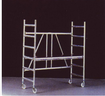
Typ KL 07-20-08 Maße: B 0,70 x L 2,10 x H 1,85 m Arbeitsbühnenfläche B 0,60 x L 2,00 m, Gewicht 35 kg, Standhöhe 0,80 m
