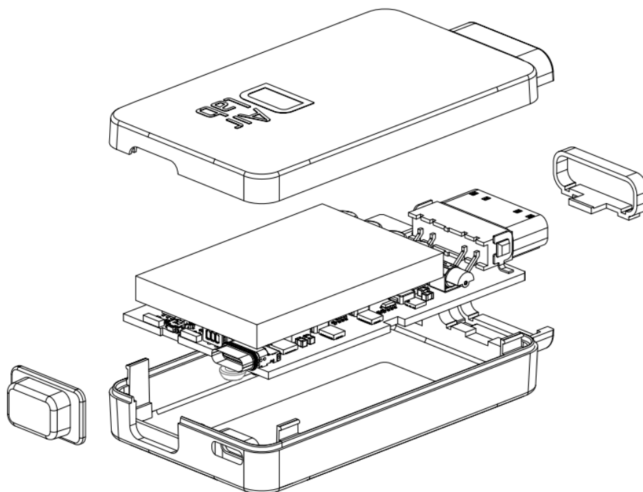
Figura 1: sistema elettronico
