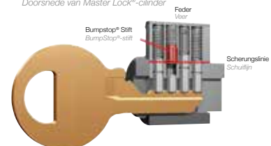
Querschnitt eines Master Lock Zylinders Doorsnede van Master Lock®-cilinder
