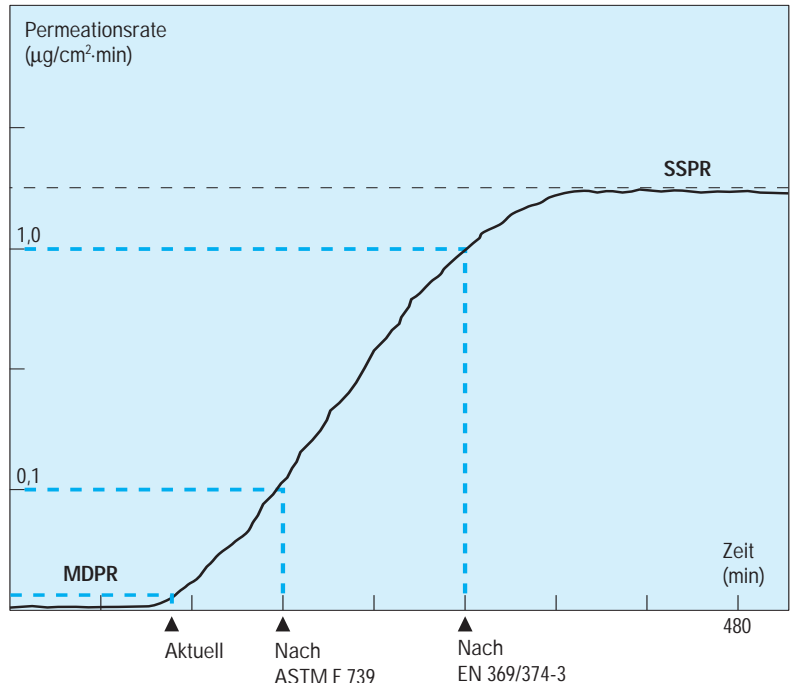
Abb. 5 Ergebnisse-Permeationsmessung
